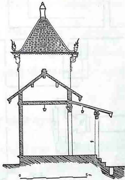
- ប្លង់ព្រះថែវព្រះវិហារព្រះកែវមរកត មាត្រដ្ឋាន ១,៥០ ' គួរដោយ លោក យូ សំអែល '
